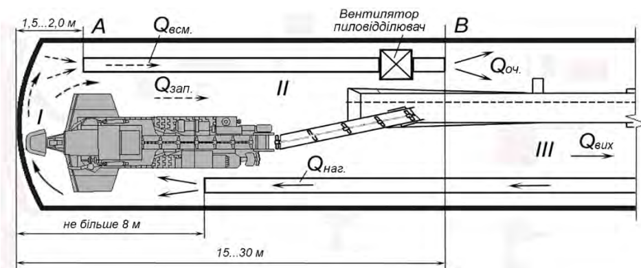
Рис. 1. Напрямок руху вентиляційних струменів при продуктивності пиловловлювача меншим, ніж витрата повітря, що подається у вибій
