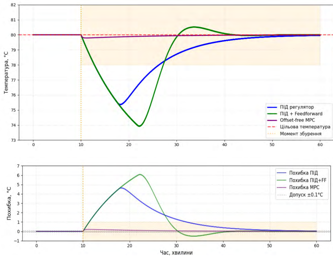
Рис. 5. Перехідні процеси різних типів регуляторів
