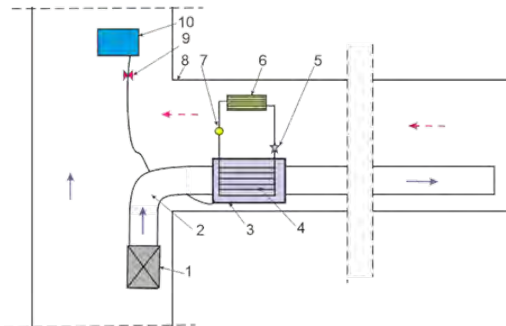
Рис. 3. Схема установки для осушения воздуха в тупиковой гірничій виробці: 1 вентилятор; 2 – повітропровід; 3 – теплоізолюваний корпус; 4 – трубчастий теплообмінник; 5 – дросель; 6 – радіатор; 7 – компресор; 8 – гірнича виробка; 9 – трубка з краном; 10 – резервуар
