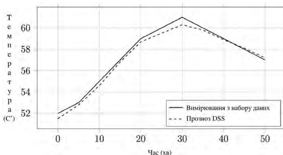
Рис. 2. Порівняння прогнозованих DSS та вимірюваних SCADA значень температури для репрезентативного сегмента трубопроводу
