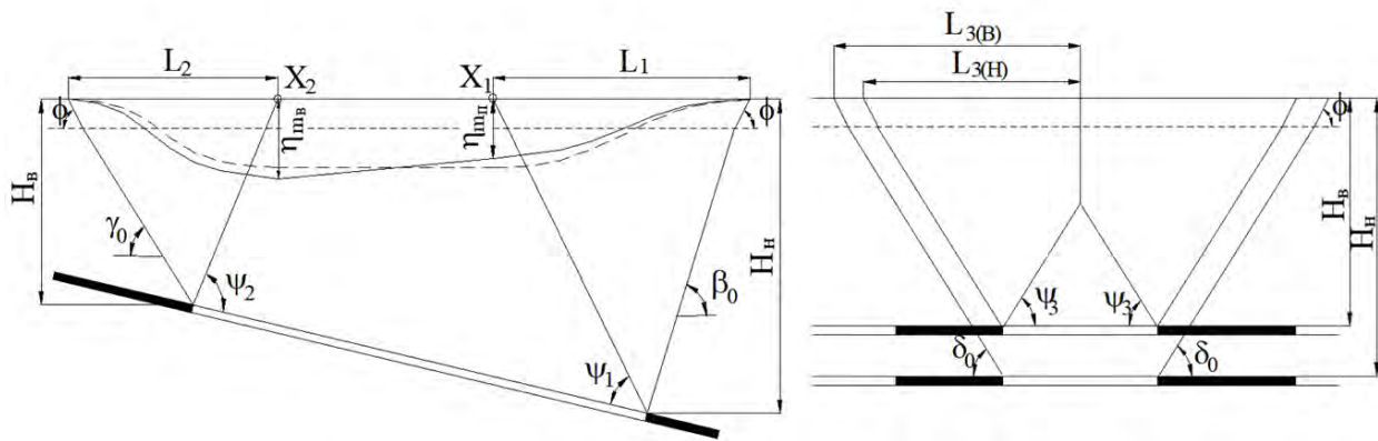
Рис. 1. Схема визначення довжин напівмудьд для випадку відпрацювання лави вхрест простягання
